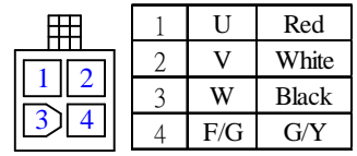
Motor Wiring
